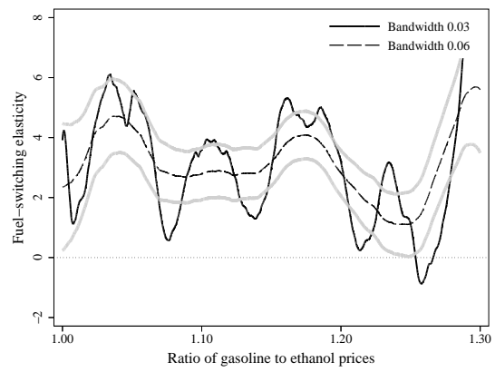
(d) Semi-parametric
